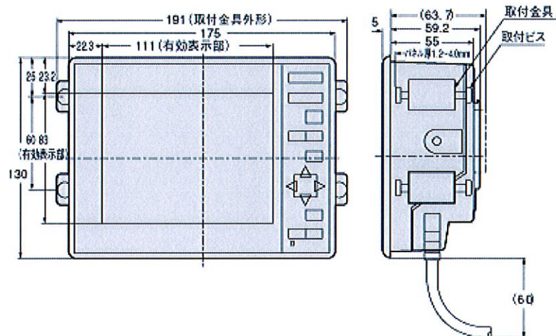
コントローラ CV-750
