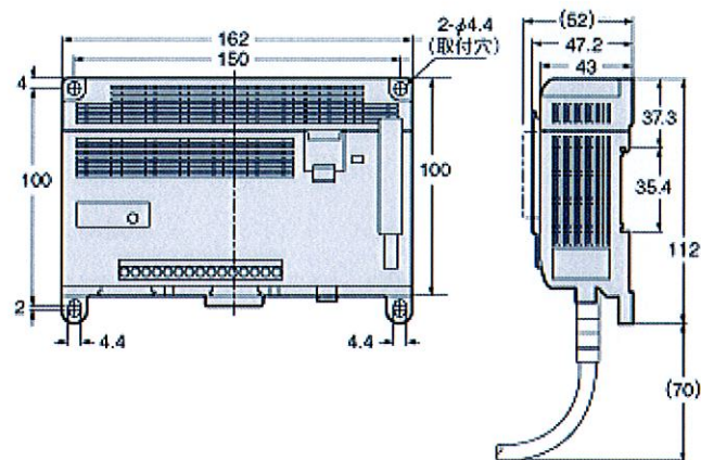
コントローラ CV-750
