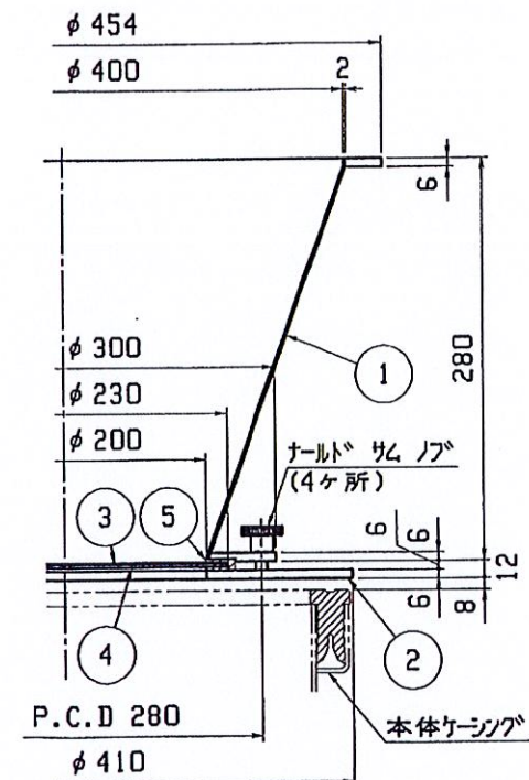
乾燥容器詳細 (S=1/4)
